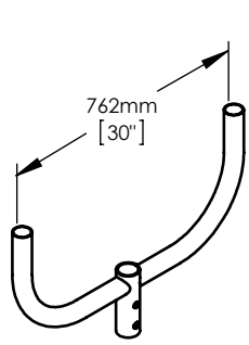
CEB-2-180°
